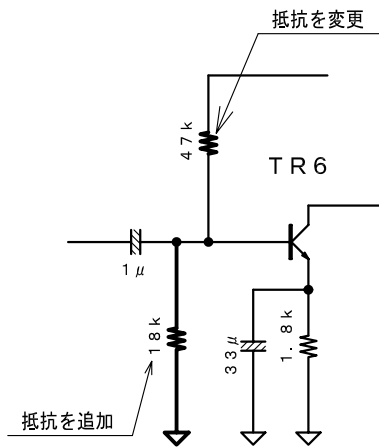
改造後回路
