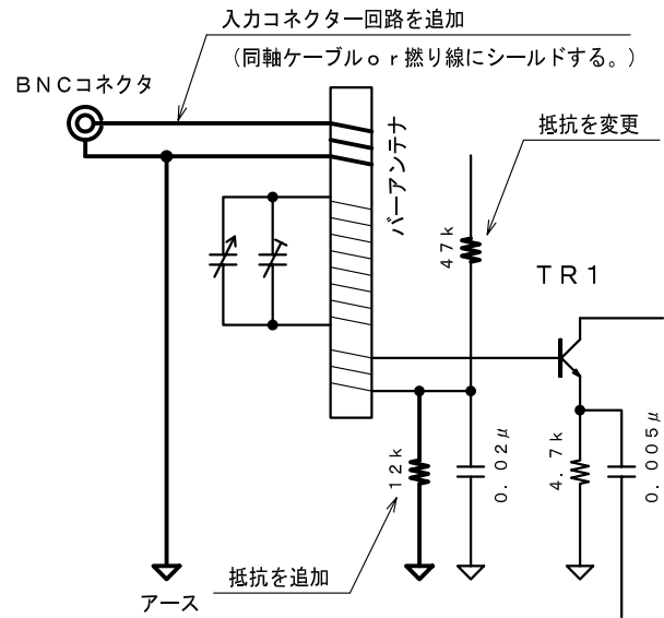
改造後回路
